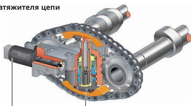
Гидравлический электромагнитный клапан
