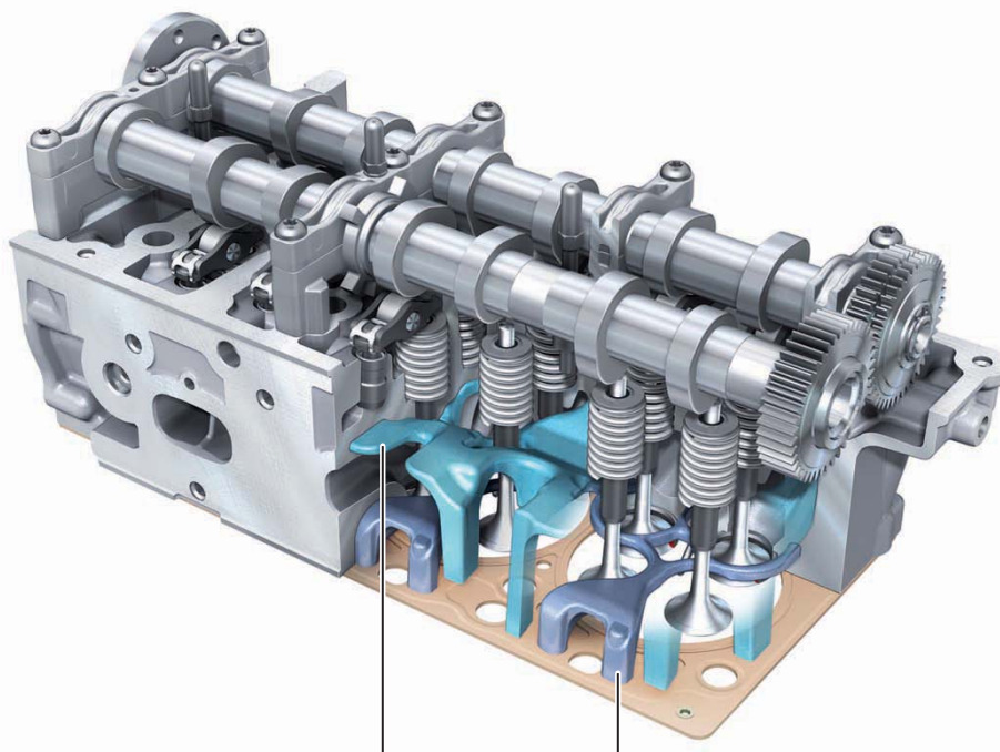
Верхний канал циркуляции ОЖ
